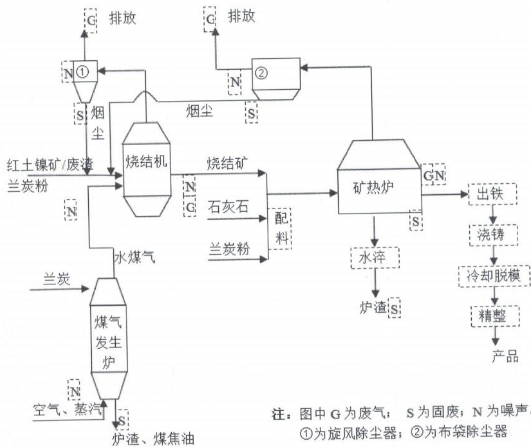
生产工艺流程及产污环节图
